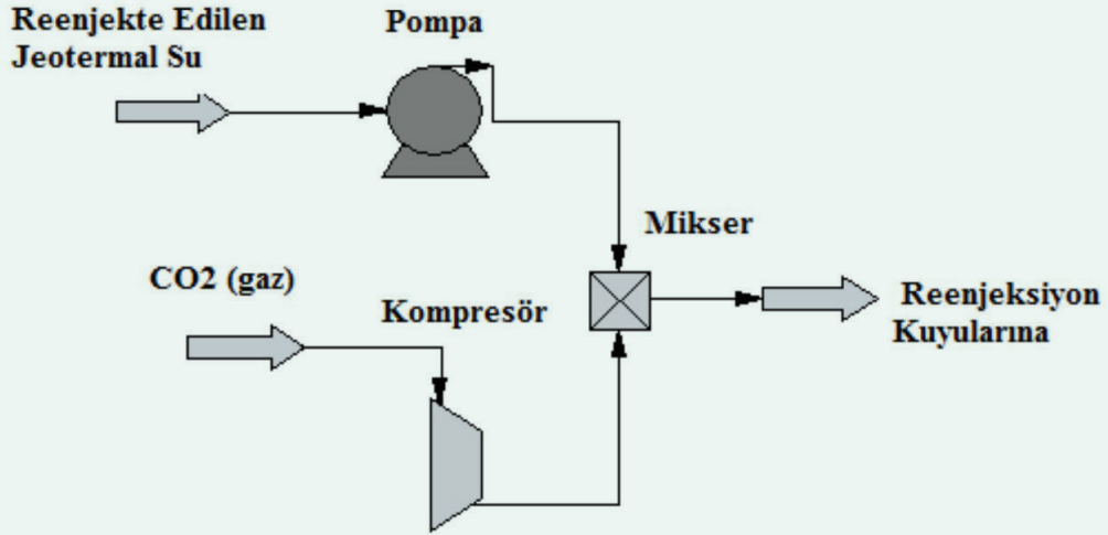
Şekil 36 | CO 2 enjeksiyon sistemi (Aksoy vd., 2017)
