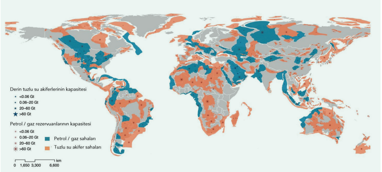
Şekil 46 | Dünya’da Karbon Depolama Potansiyel Sahaları (Wei vd., 2021)
