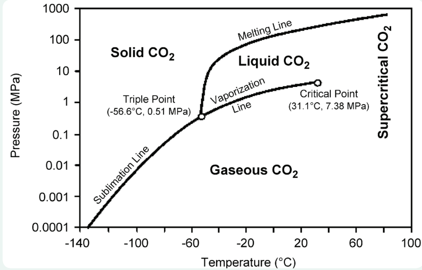
Şekil 10 | \text{CO}_2 Faz Diyagramı (Bachu vd., 2008)
